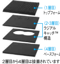
2層目から4層目は接着されています。
